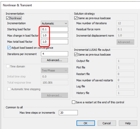
Load parameters for ramping up
